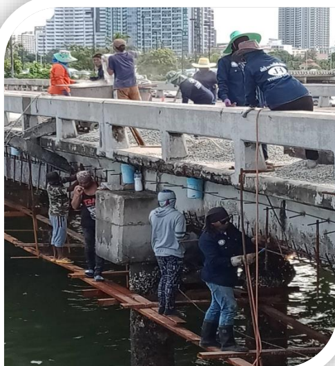
ซ่อมแซมท่าเทียบเรือเกาะลอย
